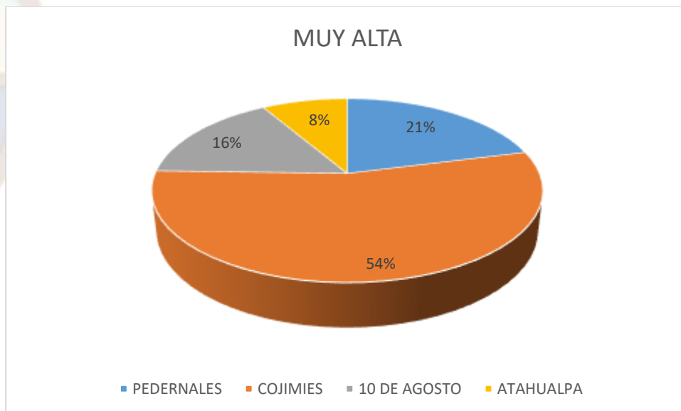
Ilustración 32.- Unidad Territorial Con Susceptibilidad De Deslizamiento Muy Alta
