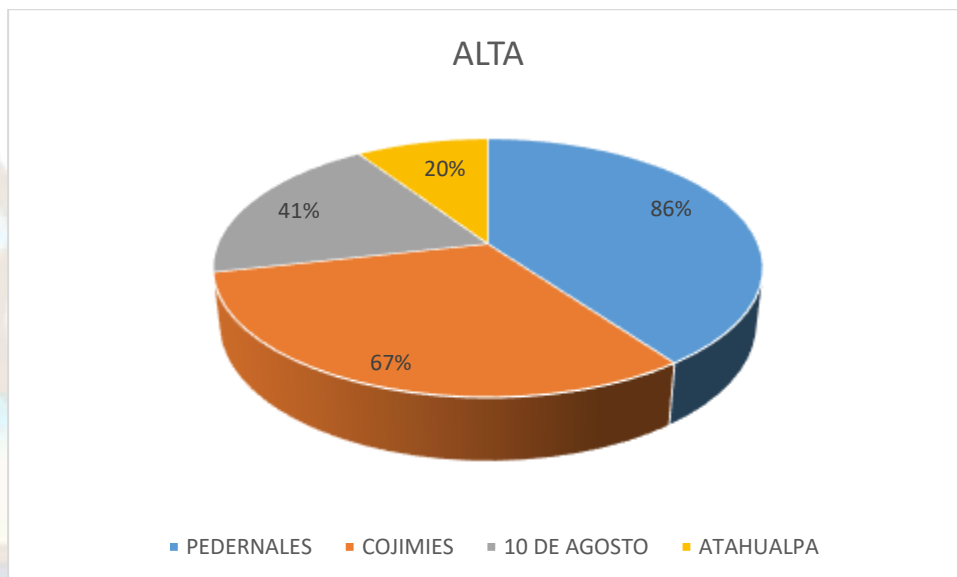
Ilustración 33.- Unidad Territorial Con Susceptibilidad De Deslizamiento Alta
