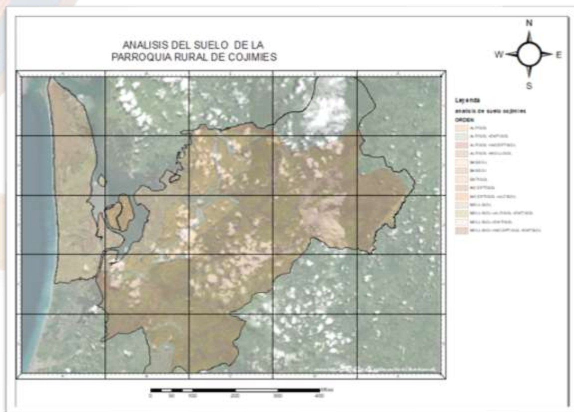
Ilustración 26.- Análisis del Suelo
