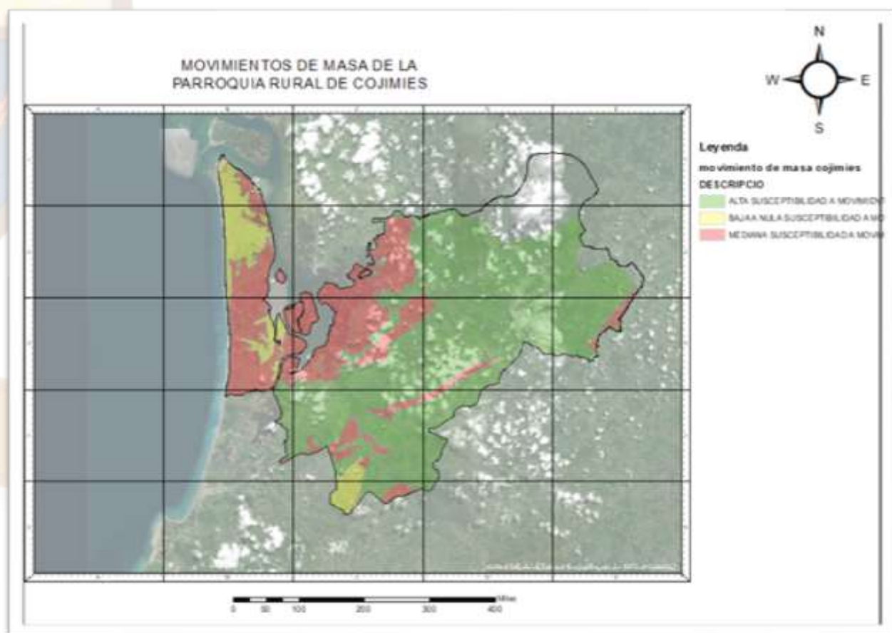
Ilustración 31.- Movimiento de Masa
